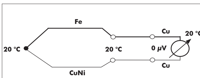
Abb. 9: Nullpunkt des Messgerätes
